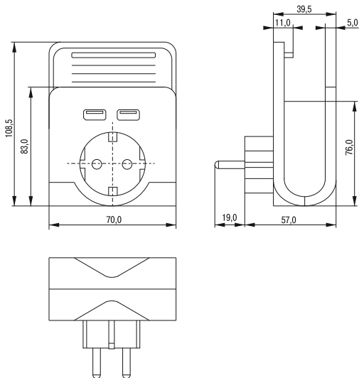
Рисунок 1 – Адаптер Т-02/01
